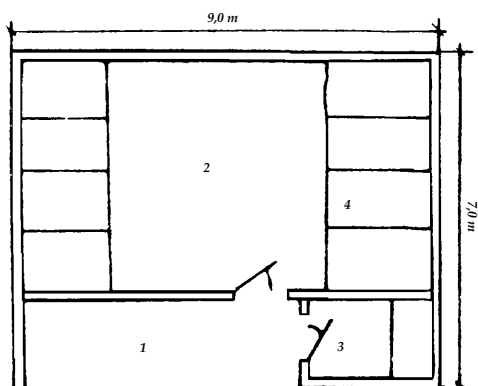
5 pav. Grūdų klėties planas:
