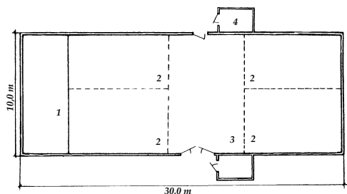
10 pav. Klojimo planas: 1 – pašiūrė (pavietis), 2 – šalinės, 3 – laitas, 4 – peludės (peludnikai)
