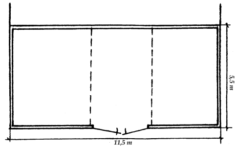
9 pav. Daržinės planas
