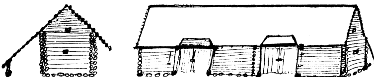
7 pav. Didžiosios daržinės piešinys (rekonstrukcija)
