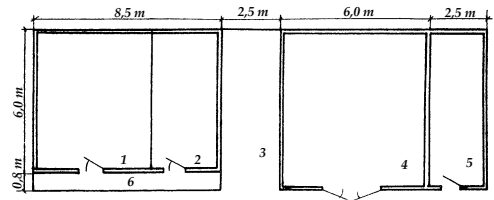
4 pav. Drabužių klėties, pašiūrės, ratinės ir tvartelio planas:
