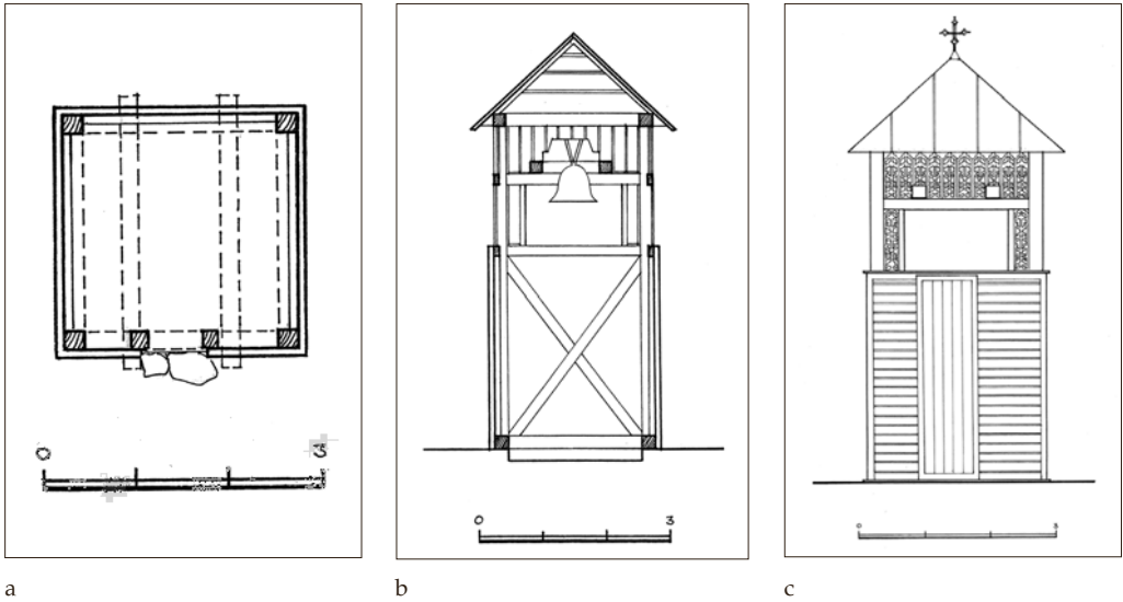
8 pav. Skapiškio varpinė: a) planas, b) pjūvis, c) pagrindinis fasadas. Sudarė A. Rupeika
