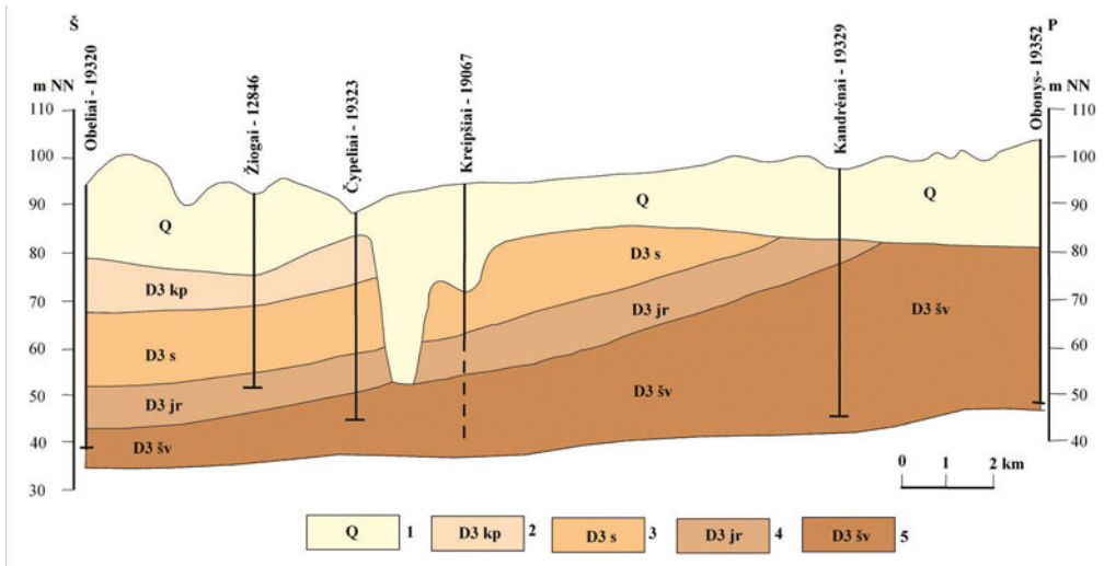
2 pav. Skapiškio valsčiaus teritorijos prekartero geologinis pjūvis (Marcinkevičius, 2014). Sutartinius ženklus žr. 1 pav.
