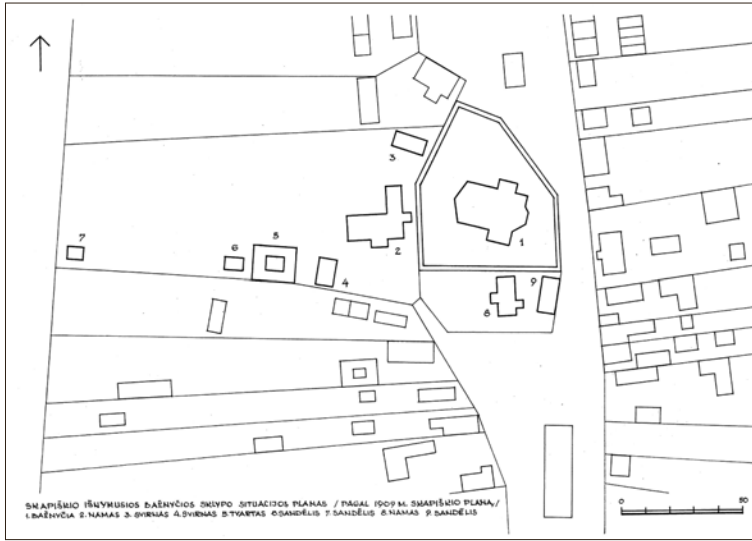
5 pav. Skapiškio išnykusios parapiinės bažnyčios ir jai priklausiusių trobesių situacijos planas. Parengė A. Rupeika pagal 1909 m. planą
