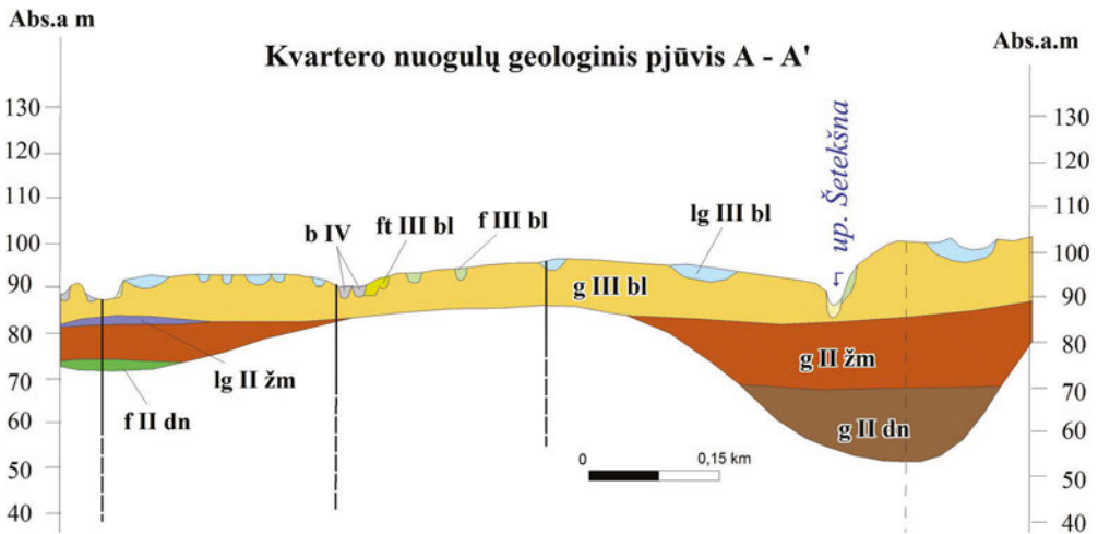
3 pav. Kvartero nuogulų geologinis pjūvis A-A' (Jusienė, 2010). Sutartiniai ženklai: bIV – durpės (nesuskirstytos), paskutiniojo apledėjimo Baltijos stadijos limnoglacialinės nuosėdos (lgIIIbl), fliuvioglacialinės nuogulos (fIIIbl), fliuvioglacialiniai ledyno pakraščio dariniai (ftIIIbl) ir glacialinės nuogulos arba morena (gIIIbl). Žemaitijos ledyno morena (gIIžm) ir limnoglacialinės nuosėdos (lgIIžm). Dainavos ledyno morena (gII dn) ir fliuvioglacialinės nuogulos (fII dn).
