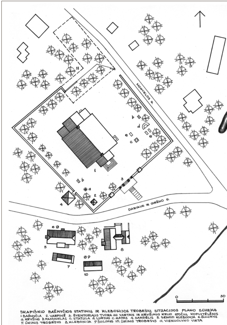
6 pav. Skapiškio bažnyčios statinių ir klebonijos trobesių situacijos plano schema. Sudarė A. Rupeika
