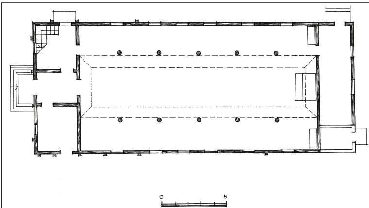
4 pav. Sintautų laikinosios bažnyčios planas. Sudarė A. Rupeika
