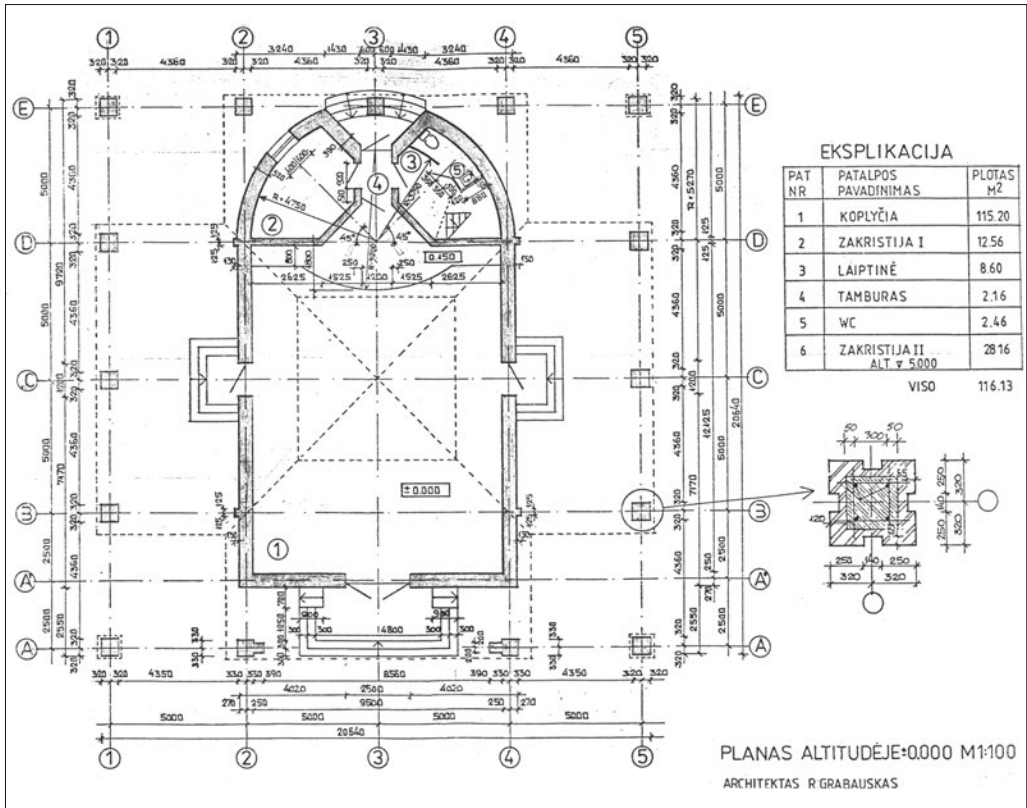
18 pav. Suodžių koplyčios planas. Projektavo archit. R. Grabauskas
