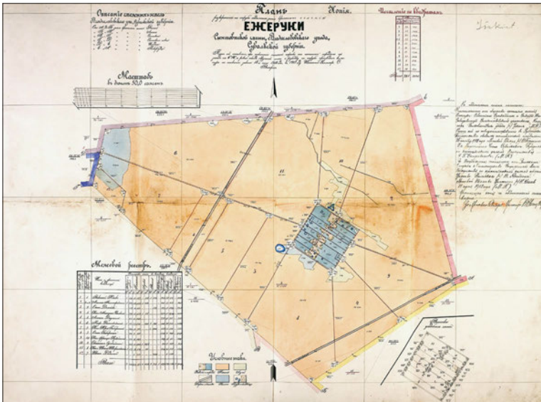
1911 m. Suvalkų gubernijos Naumiesčio apskrities Sintautų valsčiaus Ežeriūkų kaimo žemės išskirstymo į sklypus planas. Planą sudarė matininkas S. Vichertas. LCVA
