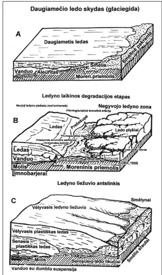
18 pav. Limnoglacialinio proceso skirtingų fazių kaita ledynmečio klimatui svyruojant (autoriaus blokdiagramos ir ledo skydo koncepcija)
