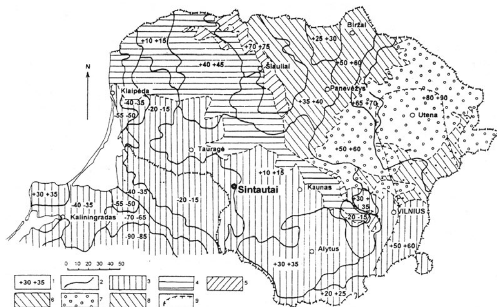
6 pav. Pokvarterinio paviršiaus pakopų ir prekvarterio sluoksnių litologinės sudėties palyginimo schema: 1 – pakopų paviršiaus absoliutinis aukštis, 2 – pakopų šlaitas, 3 – kreidos-kainozojaus uolienos (kreida, mergelis, opoka, aleuritas, smėlis), 4 – apatinio triaso ir viršutinės jūros molingos nuogulos, 5 – viršutinio permio karbonatinės uolienos, 6 – viršutinio devono karbonatinės ir molingos karbonatinės uolienos, 7 – viršutinio-vidurinio devono (Šventosios svita ir Upninkų serija) smėlingos uolienos, 8 – vidurinio devono (Narvos svita) karbonatinės ir molingos karbonatinės uolienos, 9 – neogeno aleuritinių-smėlingų nuogulų sporadinio paplitimo arealas (Šliaupa A. Ten pat, p. 46–57)
