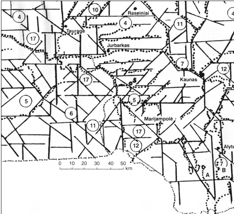
5 pav. Lūžių zonų sugretinimas su upių tinklu
