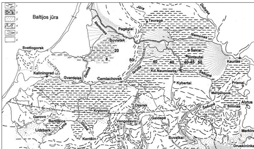
17 pav. Pietvakarių Lietuvos ir Kaliningrado srities ledyno pakraštinių darinių, limnoglacialinių ir smėlinių lygumų žemėlapis (P. Vaitiekūnas, 1972, su nedideliais autoriaus papildymais)
