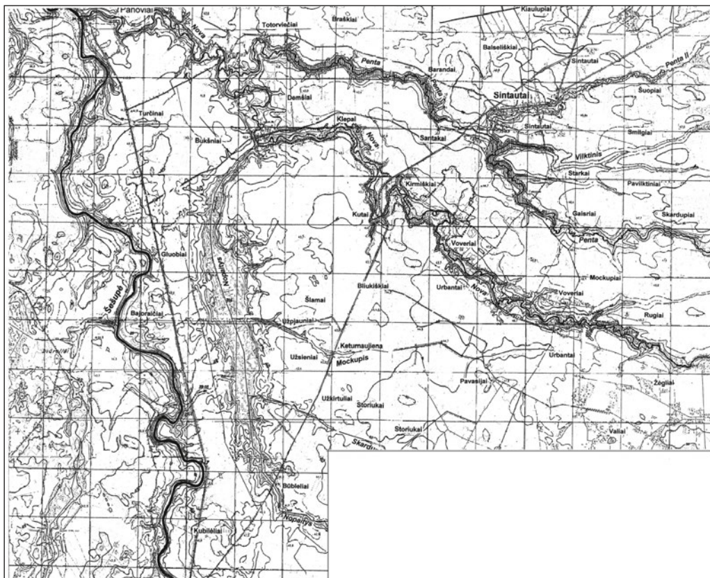
25 pav. Novos, Nopaičio ir Pentos žemupių slėnių morfometrija ir Šešupės slėnis tarp Kubilėlių ir Panovių. Užbrūkšniuoti 2 Pentos tvenkiniai, o taškais pažymėtas Novos hidrografinis draustinis
