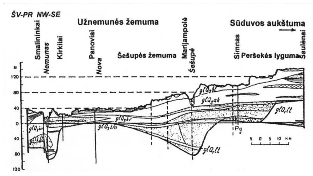
8 pav. Kvartero (ledynmečio nuogulų) profiliai per Užnemunės lygumą (V. Vonsavičius, 1973). Indeksų reikšmes žr. 9 pav.
