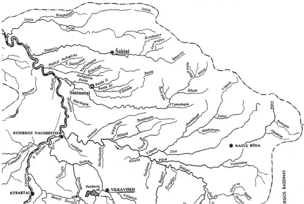
24 pav. Užnemunės lygumos Šešupės vidurupio upynas
