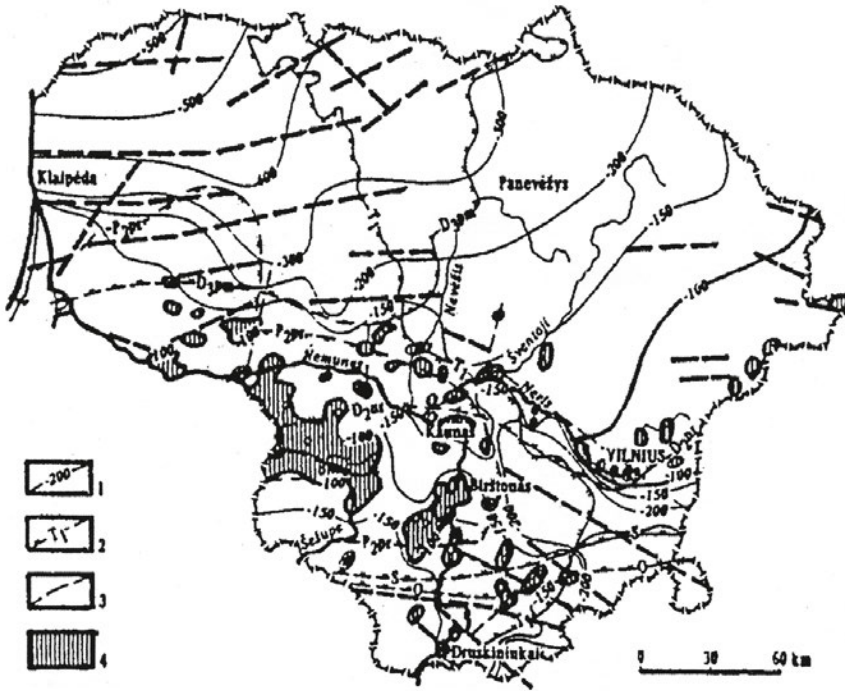
23 pav. Židininės hidrogeocheminės anomalijos, susidariusios mineralizuotam vandeniui srūvant iš gilumos (pagal Z. Šontą, 1972). 1 – požeminio vandens, turinčio daugiau kaip 350 mg/l chloro, slūgsojimo gylio izohipsė, m, 2 – regioninių vandensparų paplitimo riba ir jų geologinis indeksas, 3 – tektoniniai lūžiai, 4 – injekcinio tipo židininės hidrogeologinės anomalijos
