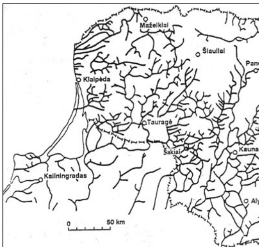
22 pav. Pokvarterinio paviršiaus reljefo pobūdis ir senieji palaidoti įrežiai bei upių slėniai. Tai svarbiausios įrežių sistemos, kai kur besikūrusios visą kvartero epochą nuo pat neogeno periodo (sistemos); A. Šliaupa, 1997
