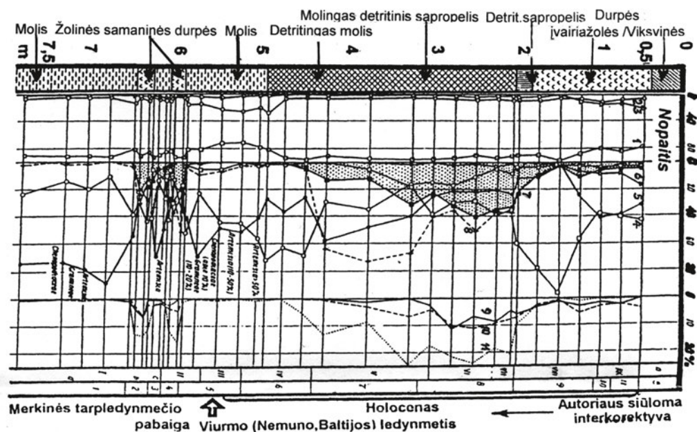
27 pav. Pelkės vidurio gręžinys ir žiedadulkių diagrama. Diagramos ženklai: 1 – medžiai, 2 – žolės, 3 – sporiniai augalai, 4 – beržas, 5 – eglė, 6 – pušis, 7 – plačialapiai med., 8 – lazdynas, 9 – ažuolas, 10 – liepa, 11 – guoba. 1–12 ir I–X-holoceno klimatinis periodizavimas
