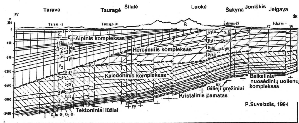
3 pav. Geologinis tektoninis PV–ŠR krypties profilis, rodantis skirtingo giluminių jėgų poveikio ir sąskaidos kompleksus (P. Suveizdis, 1994). Sistemų indeksai: Q – koartero, N – neogeno, P – paleogeno, K – kreidos, J – jūros, T – triaso, P – permo, D – devono, S – silūro, O – ordoviko, E – kambro, V – prekambro, vėndo kompl.
