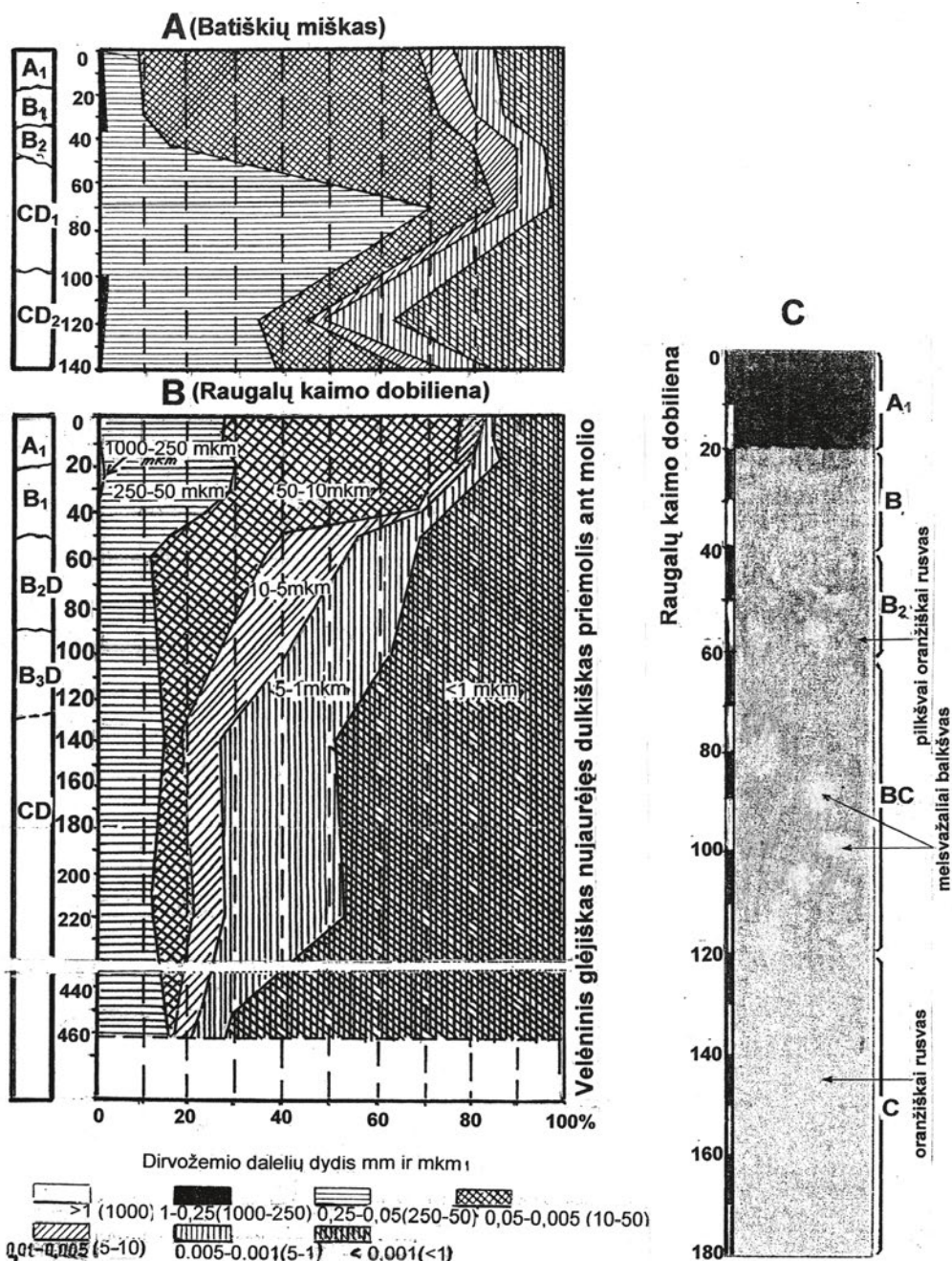
37 pav. Būdingiausių derlingųjų lygumos dirvožemių, paliestų jaurėjimo, velėnėjimo ir glėjėjimo procesų, profiliai. Dirvožemio dalelių dydžio ir spalvos kaita prakasoje (J. Buloto tyrimų medžiaga, 1953, 1961, 1965)
