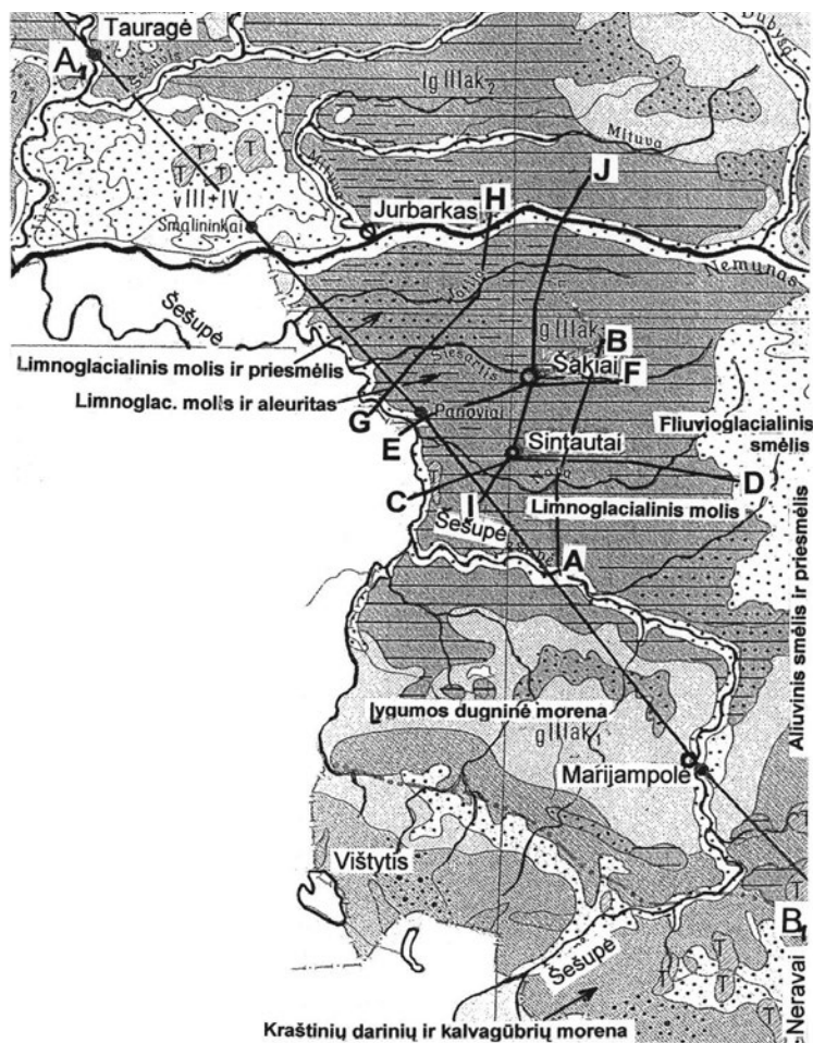
10 pav. Kvartero didžiojo profilio ir Užnemunės lygumos vietinių profilių vietos
