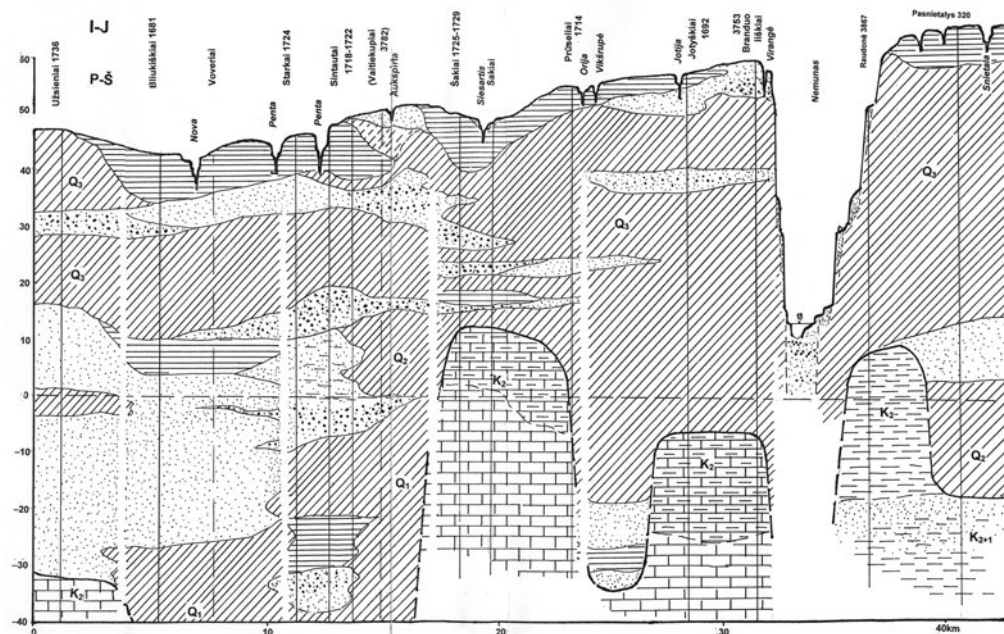
15 pav. Platuminis kvartero profilis per Sintautų, Šakių apylinkes ir panemunę I-J (R. Kuskas)
