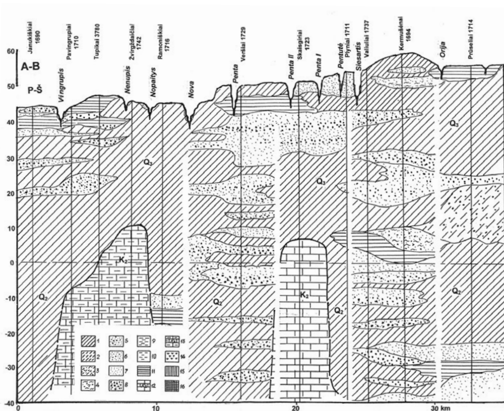
11 pav. Platuminis kvartero dangos profilis A–B per Užnemunės lygumą (sudarė R. Kunskas)
