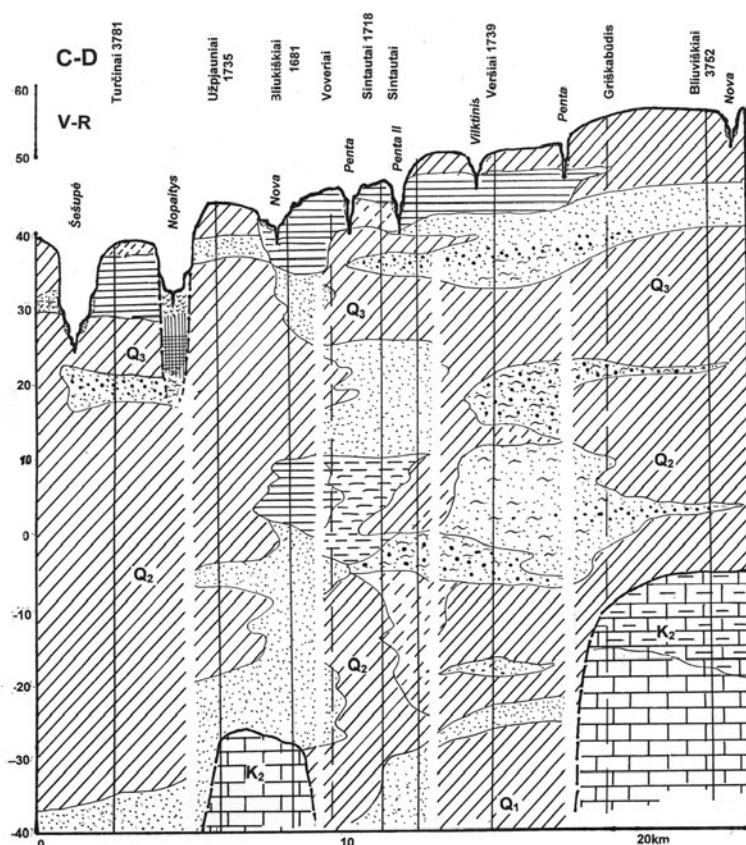
12 pav. Ilguminis koartero dangos profilis C–D per Sintautų apylinkę (R. Kunskas)
