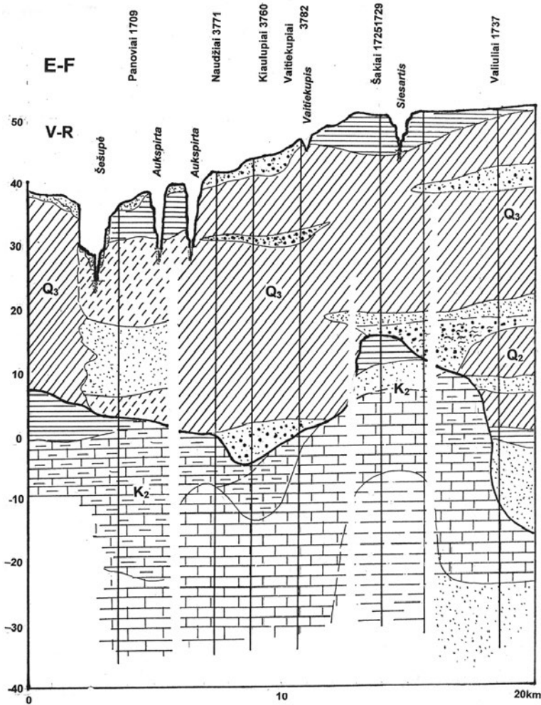
13 pav. Ilguminis kvartero dangos profilis E-F per Šakius (R. Kunskas)
