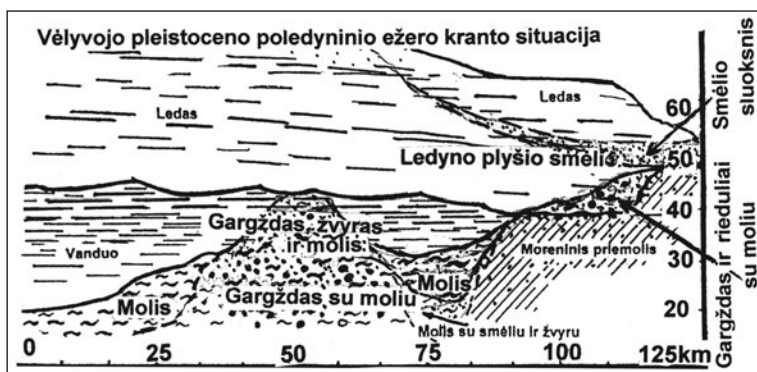
19 pav. Poledinio ežero kranto situacijos profilis pagal autoriaus koncepciją
