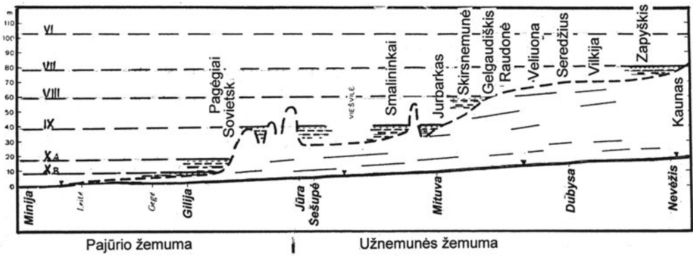
30 pav. Nemuno žemupio upėkrinta (išilginis profilis), svarbiausių 4 terasų ruožai ir ledyninių ežerų atžymėti lygiai (A. Basalykas, 1965; VI-X žymėjimai – prieledyninių ežerų kritimo etapai pagal A. Basalyką)
