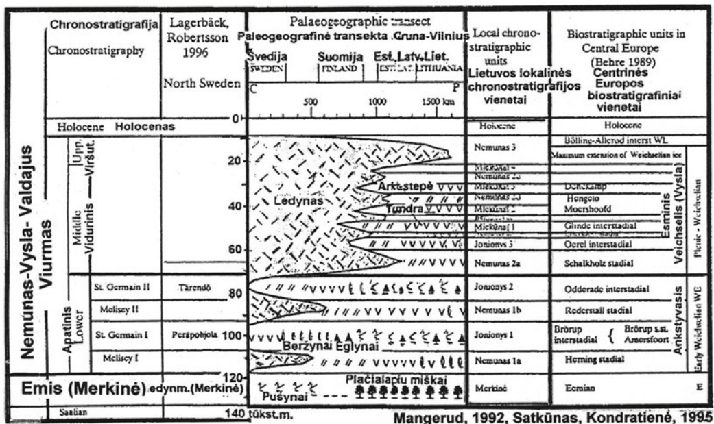
16 pav. Vėlyvojo ledynmečio Nemuno–Vyslos stratigrafijos ir paleogeografijos lentelė (Mangerud, 1992; Satkūnas, Kondratienė, 1995)
