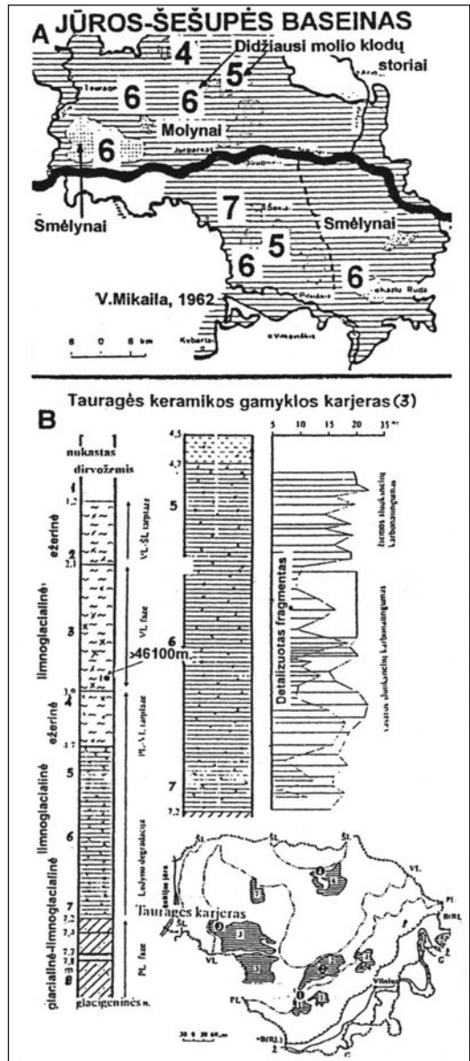
21 pav. A. Užnemunės ir Karšuvos lygumų limnoglacialiniai molynai, jų periferijoje ir iš dalies viršuje slūgsantys smėlynai, paveikti vėjo pūstymų. Skaičiai rodo didžiausią molio storį (V. Mikaila, 1962). B. Molio su priemoliu ir juostuotojo molio dvisluoksnis 6 m klotas Tauragės molyno karjere. Apatinė juostuotojo molio dalis analizuota chemiškai (A. Gaigalas, V. Dvareckas, V. Kazakauskas, 2001)
