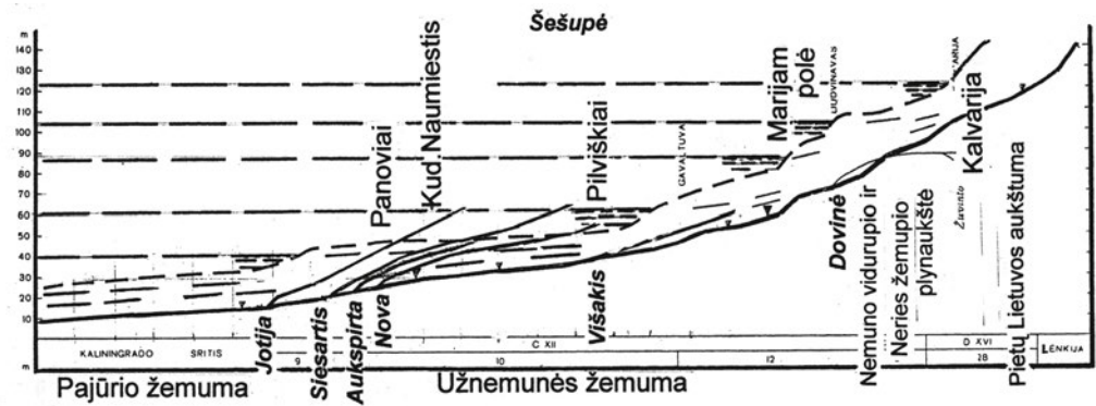
31 pav. Šešupės ir jos intakų upėkrintos
