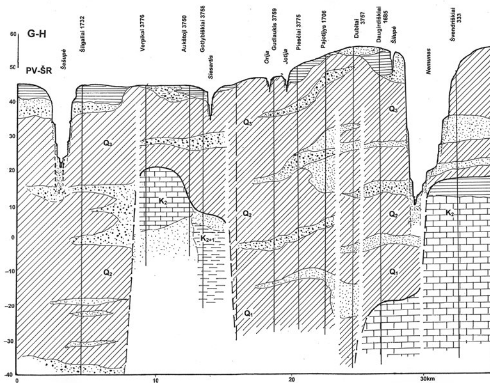
14 pav. Kvartero profilis per pašešupį ir panemunę G-H (R. Kuskas)
