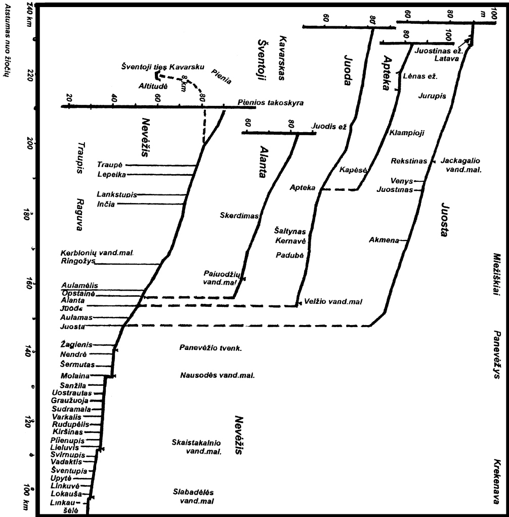
7 pav. Nevėžio aukštupio ir jo svarbesnių intakų išilginiai profiliai
