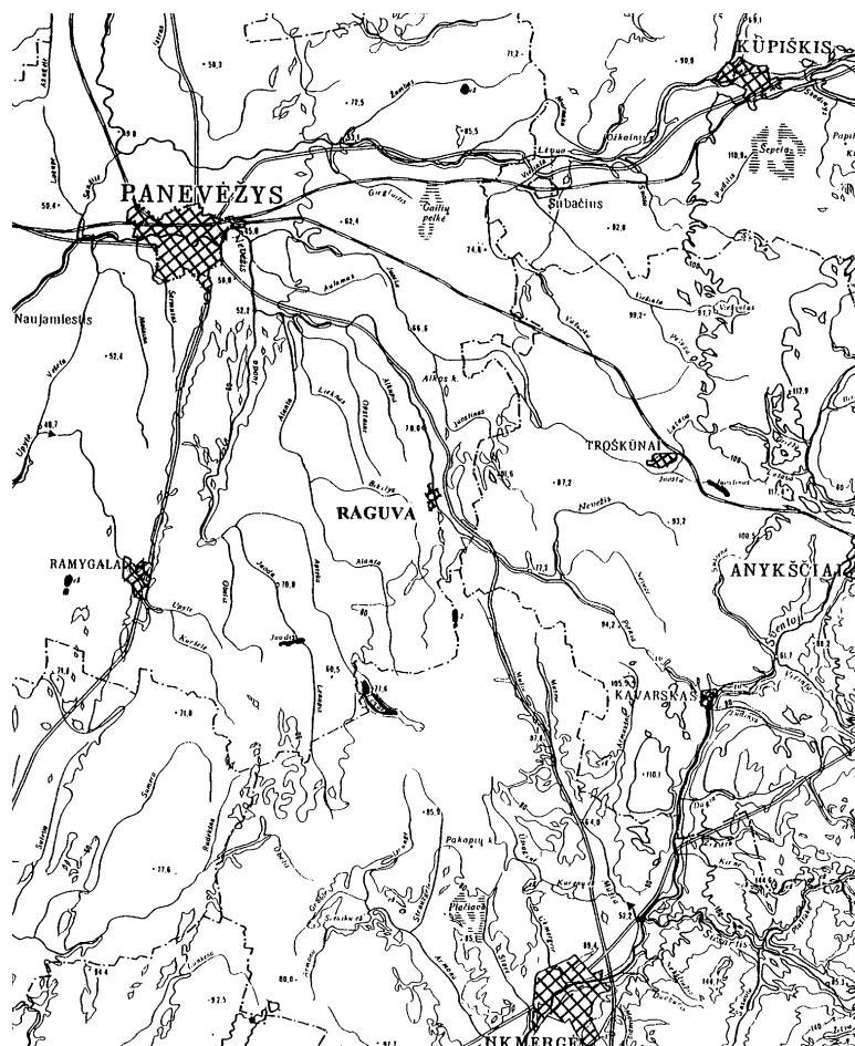
1 pav. Šiaurrytinės Nevėžio lygumos dalies reljefas. Lietuvos reljefo žemėlapis 1:300 000, išleisto Respublikos žemėtvarkos projektavimo instituto 1988 m., fragmentas
