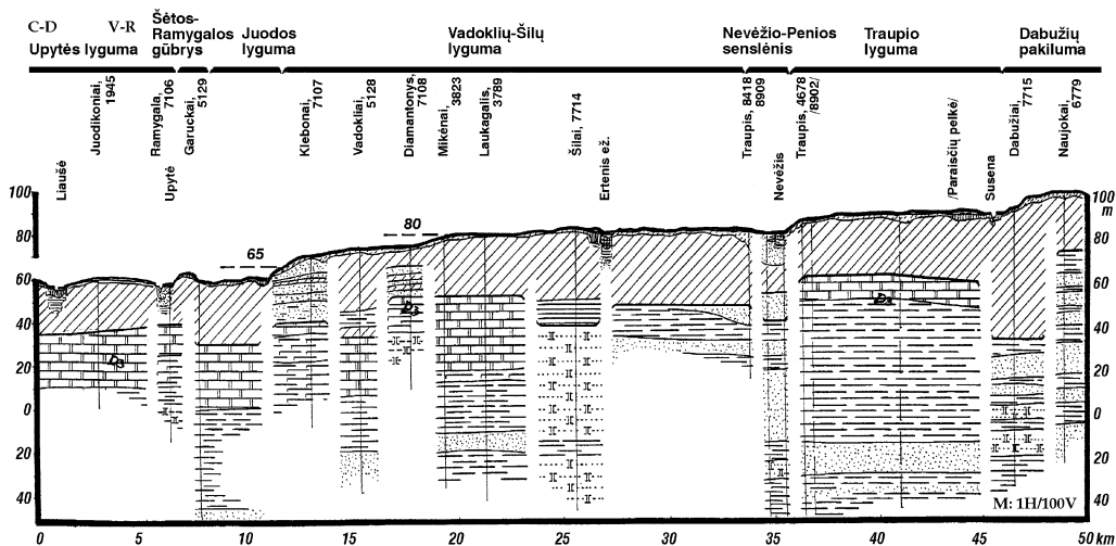
3 pav. Geologinis profilis Ramygalas–Šilai–Dabužiai. Sudarė R. Kunskas
