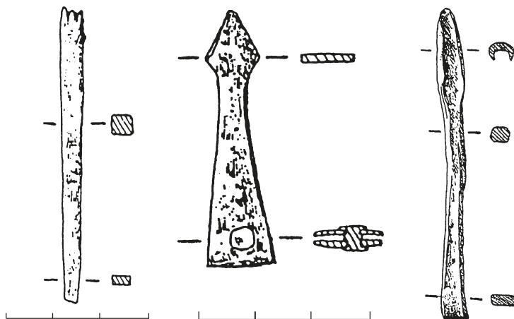
58 pav. Geležinis gražtelis, skirtas kaului ir ragui ornamentuoti, rastas Žemutiniame mieste kauladirbio sodyboje
