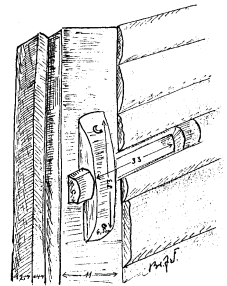
J. Kušlio gyvenamojo namo durų užraktas
