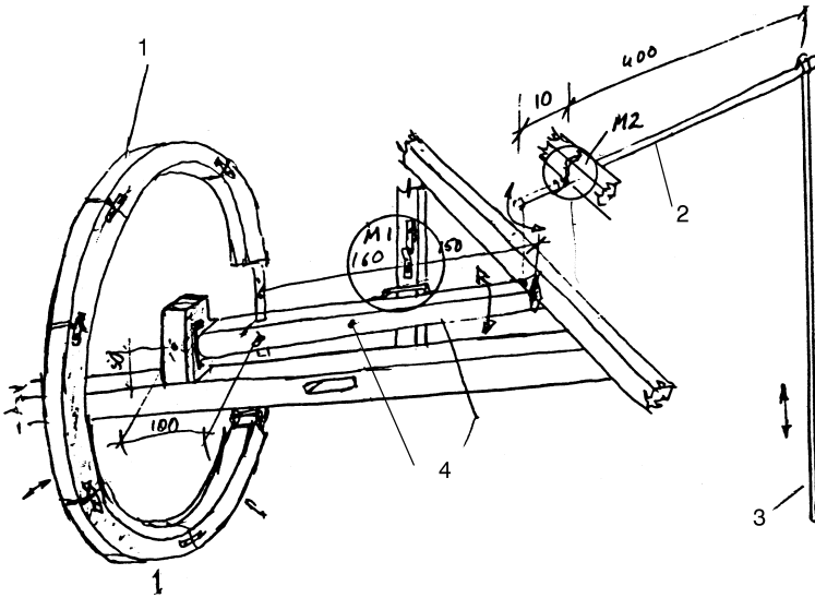
4 pav. Stabdymo mechanizmas. Piešė E. J. Morkūnas. 1 – sparninio veleno stabdymo juosta, 2 – kartelė, 3 – virvė arba grandinė, 4 – „meška“
