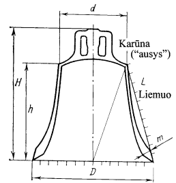
5 pav. Varpo skersinis pjūvis.
