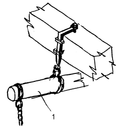
6 pav. Kartelės pakabinimo mazgas. Piešė E. J. Morkūnas. 1 – kartelė
