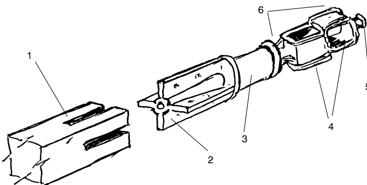
3 pav. Ketinė sparninė kryžma. Piešė E. J. Morkūnas. 1 – veleno išdrožas, 2 – „uodega“, 3 – kaklas, 4 – posparnių įtvėrimo vieta, 5 – spurgas, 6 – „galva“
