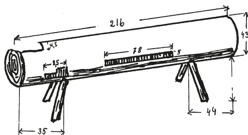
15 pav. Darbatalis. 2001 m. Matavo ir braižė Elvyra Straševičienė
