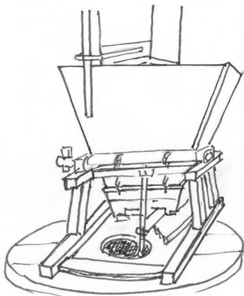
Grūdų bėrimo į gornas mechanizmas. 2002 m. E. J. Morkūno piešinys
