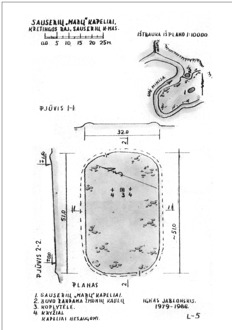
Prystovų k. (neteisingai plane nurodyta Sauserių k.) senųjų kapinių planas. Sudarė Ignas Jablonskis, 1986 m.
