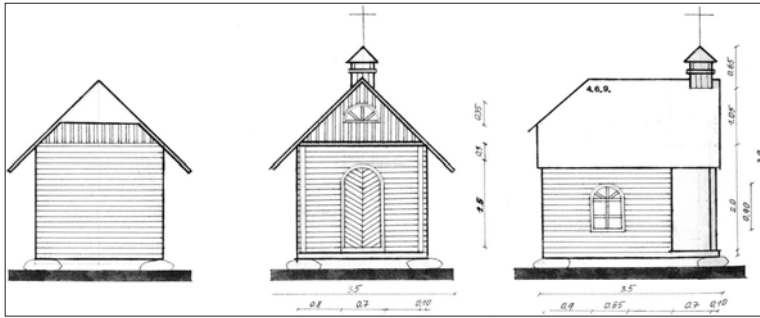
R. Čekėnaitės diplominio darbo „Pakutuvėnų Kryžiaus kelio stotys“ planas: 4-osios stoties „Jėzus susitinka savo Motiną“ brėžinys (kopija)
