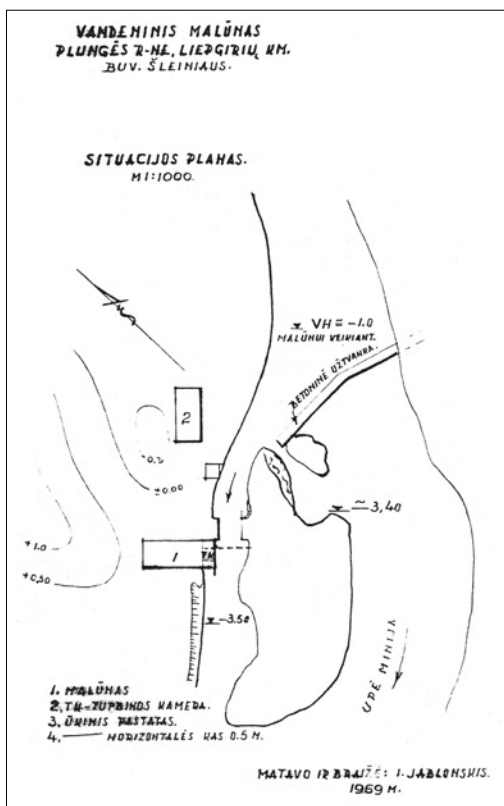
Liepgirių kaimo Šleiniaus vandens malūno situacijos planas. Braižė Ignas Jablonskis, 1969 m.
