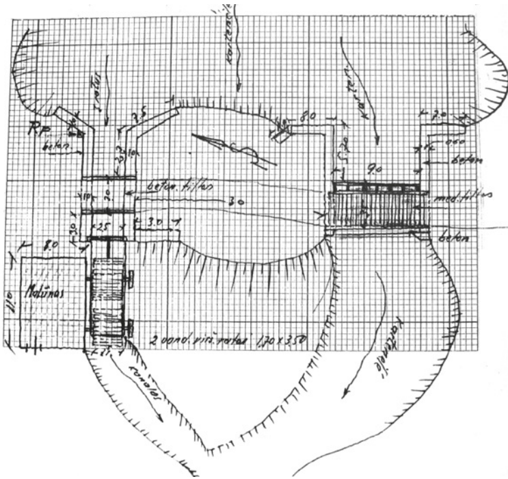
Užtvankos su malūnu ant Kartenalės situacijos schema. Apie 1936 m. Kopija iš E. J. Morkūno rinkinio
