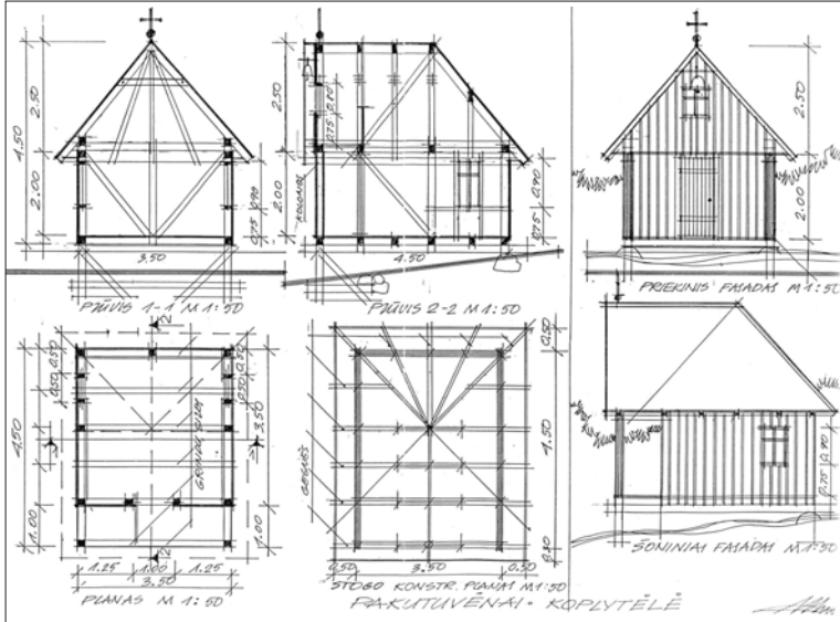
7-osios Kryžiaus kelio stoties „Jėzus parpuola antrą kartą“ koplyčios brėžinys. 1996 m. Archit. Jonas Mockus (Plateliai). Rimos Čekėnaitės asm. archyvas (kopija)
