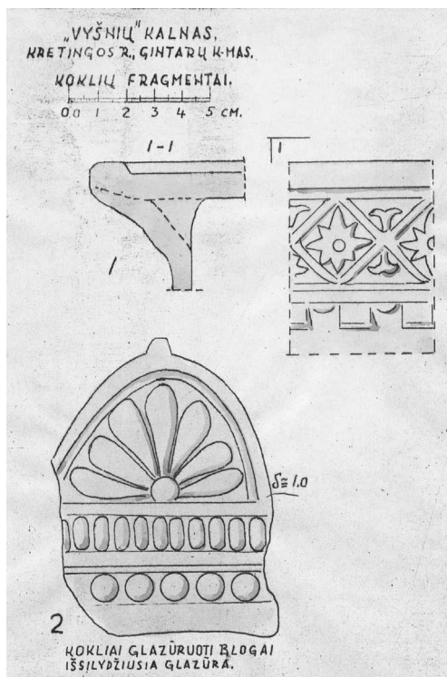
Gintarų k. dvarvietėje, vad. Vyšnių kalnu, rastų koklių fragmentai. 1987 m. Braižė I. Jablonskis
