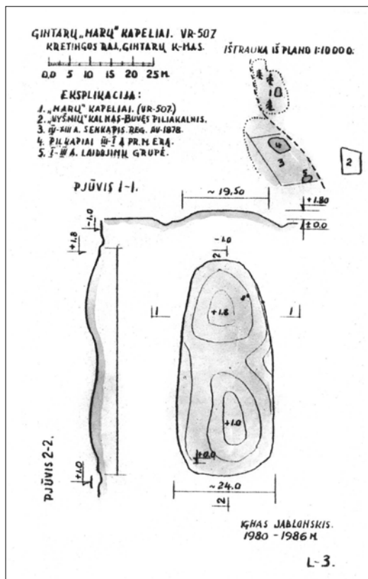
Gintarų k. senųjų kapinių planas. Sudarė Ignas Jablonskis, 1986 m.
