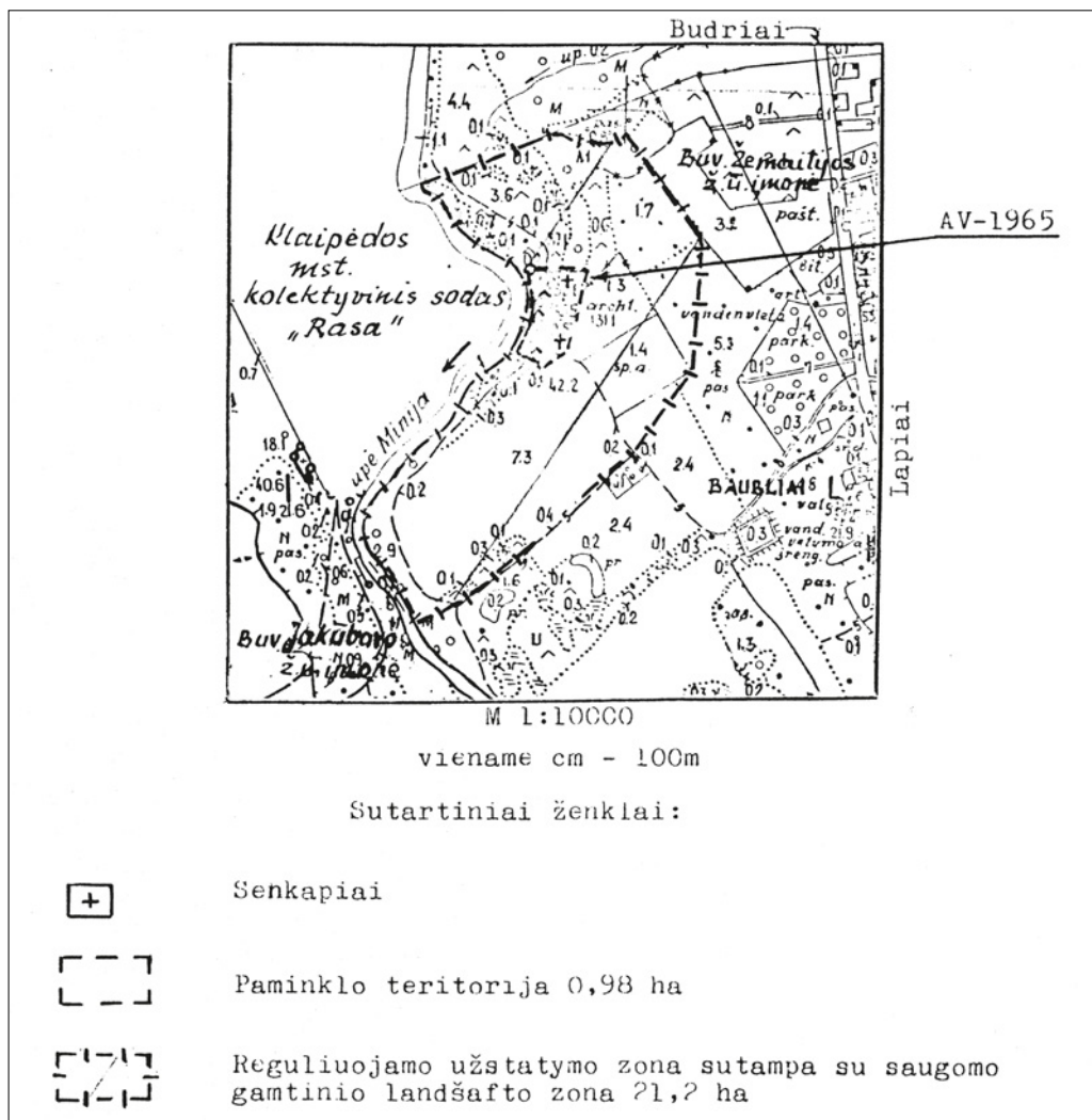
Baublių pilkapių situacijos schema. Sudarė Aldona Rutkauskienė, 1992 07 24
