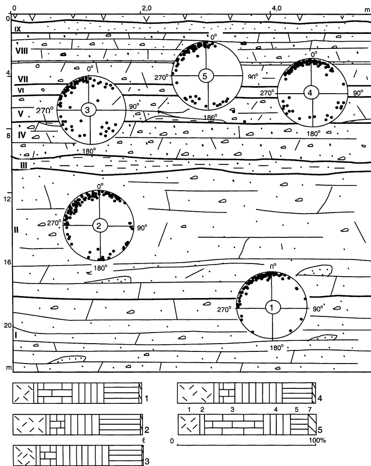
2 pav. Morenų smulkaus gargždo petrografinė sudėtis (integralinės diagramos) ir orientacija (taškinės diagramos) Alanto upės atodangoje Gintarų kaimo apylinkėse.
