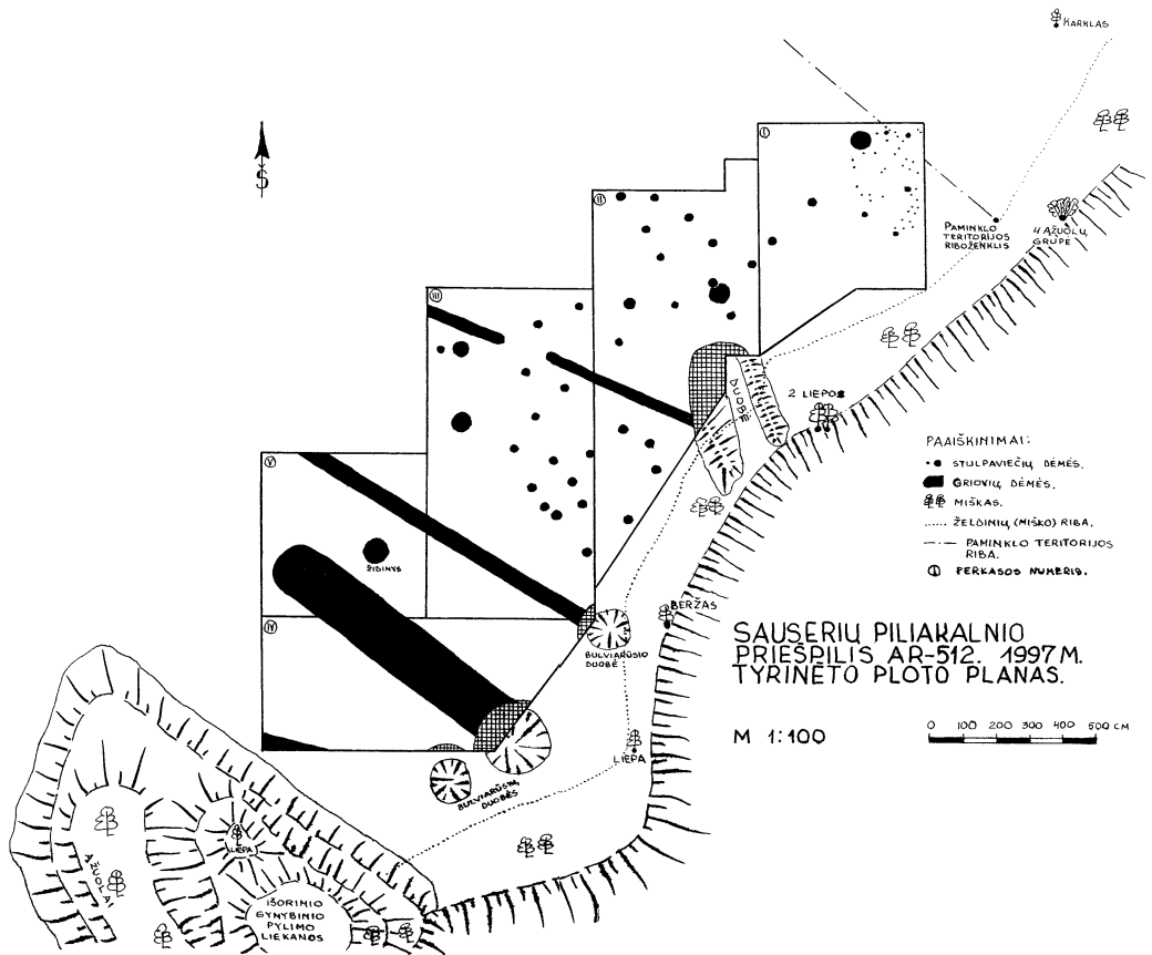
Sauserių piliakalnio priešpilio 1997 m. tyrinėto plogo planas. 1997 m. Sudarė J. Kanarskas
