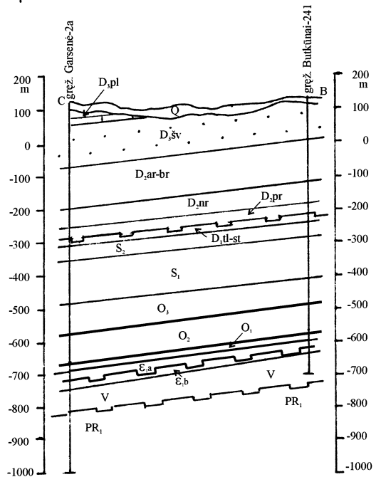
5 pav. Geologinis pjūvis B–C (gręžinys Butkūnai-241–Garsenė-2a). Sutartiniai ženklai 3 ir 4 pav.
