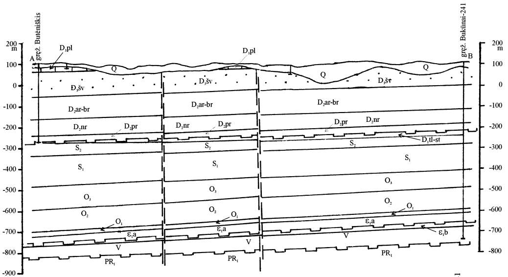
4 pav. Geologinis pjūvis A–B (gręžinys Butėniškis–Butkūnai-241): 1 – struktūrinių kompleksų riba; 2 – geologinių sluoksnių riba.
