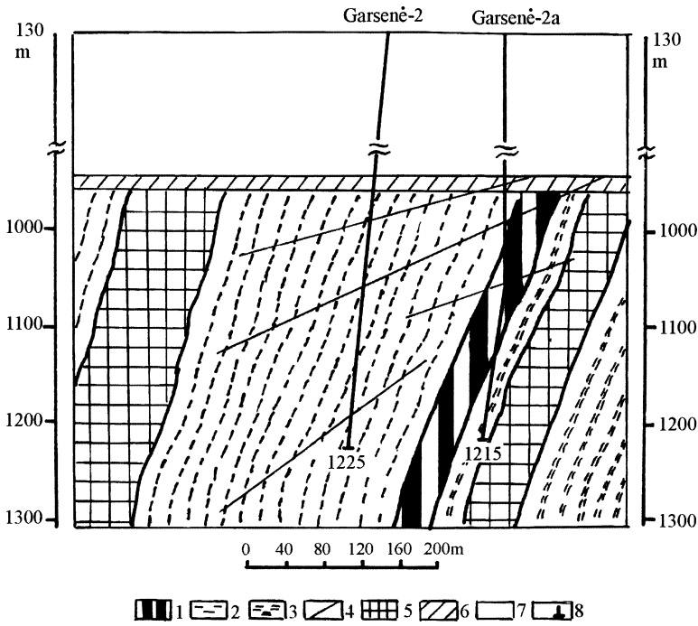
6 pav. Geologinis pjūvis per Tumasonių magnetinę anomaliją ir režinius Garsenė-2 ir Garsenė-2a 13 : 1 – kvoarcitinis magnetitas, magnetitinis kvarcitas, kvarcinis amfibolinis magnetitas; 2 – biotitinis gneisas ir migmatitinis plagiogranitas; 3 – biotitinis-albitinis gneisas; 4 – lūžiai; 5 – geležies rūdos kūnai, numatomi pagal magnetinio lauko tyrimus gręžiniuose; 6 – kristalinio pamato uolienų dūlėjimo pluta; 7 – gręžinys, jo numeris ir gylis
