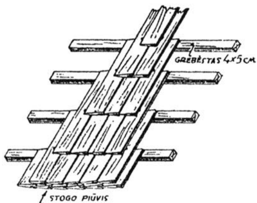
Trijų sluoksnių malksnų stogas.
