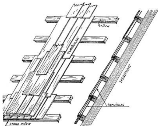
Trijų sluoksnių skiedrų stogas. Apatinį sluoksnį vadino pamušalu, pamušaliniu.
