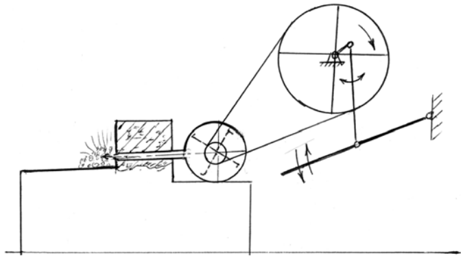
Rankena sukamas ventilatorius orui įpūsti į žaizdą
