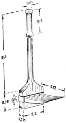
Rankinis karštuvas
