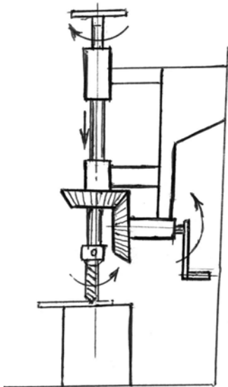
Rankena sukamos metalo grėžimo staklės
