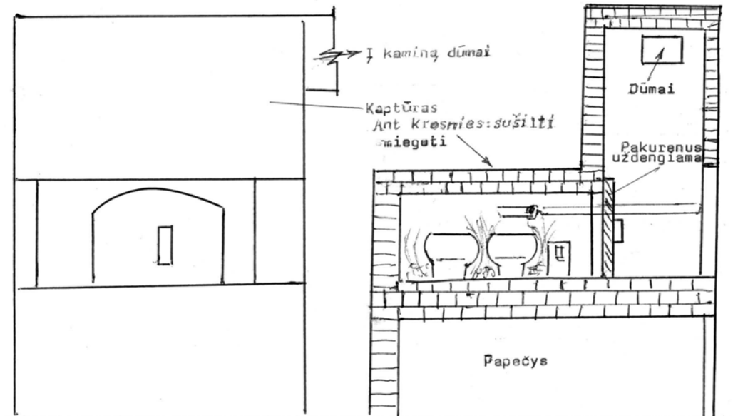
Kaimo krosnis
