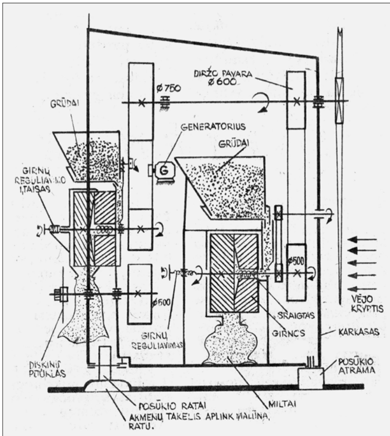
3 pav. Malūno mechanizmų schema po rekonstrukcijos
