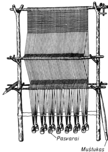
Muštukas
