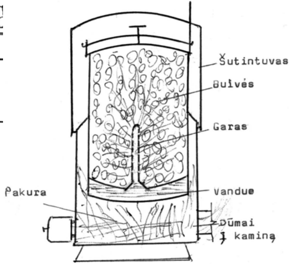
Šutintuvas
