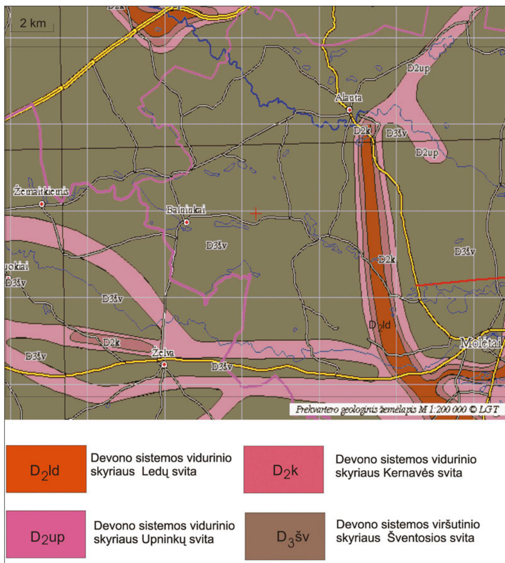
1 pav. Geologinis žemėlapis
