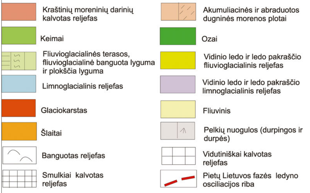
3 pav. Geomorfologinis žemėlapis
