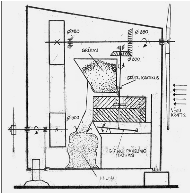
2 pav. Malūno mechanizmų schema iki 1949 m.
