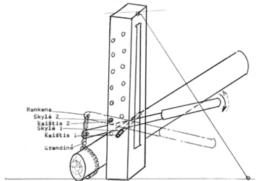
Rąstų keltuvas
