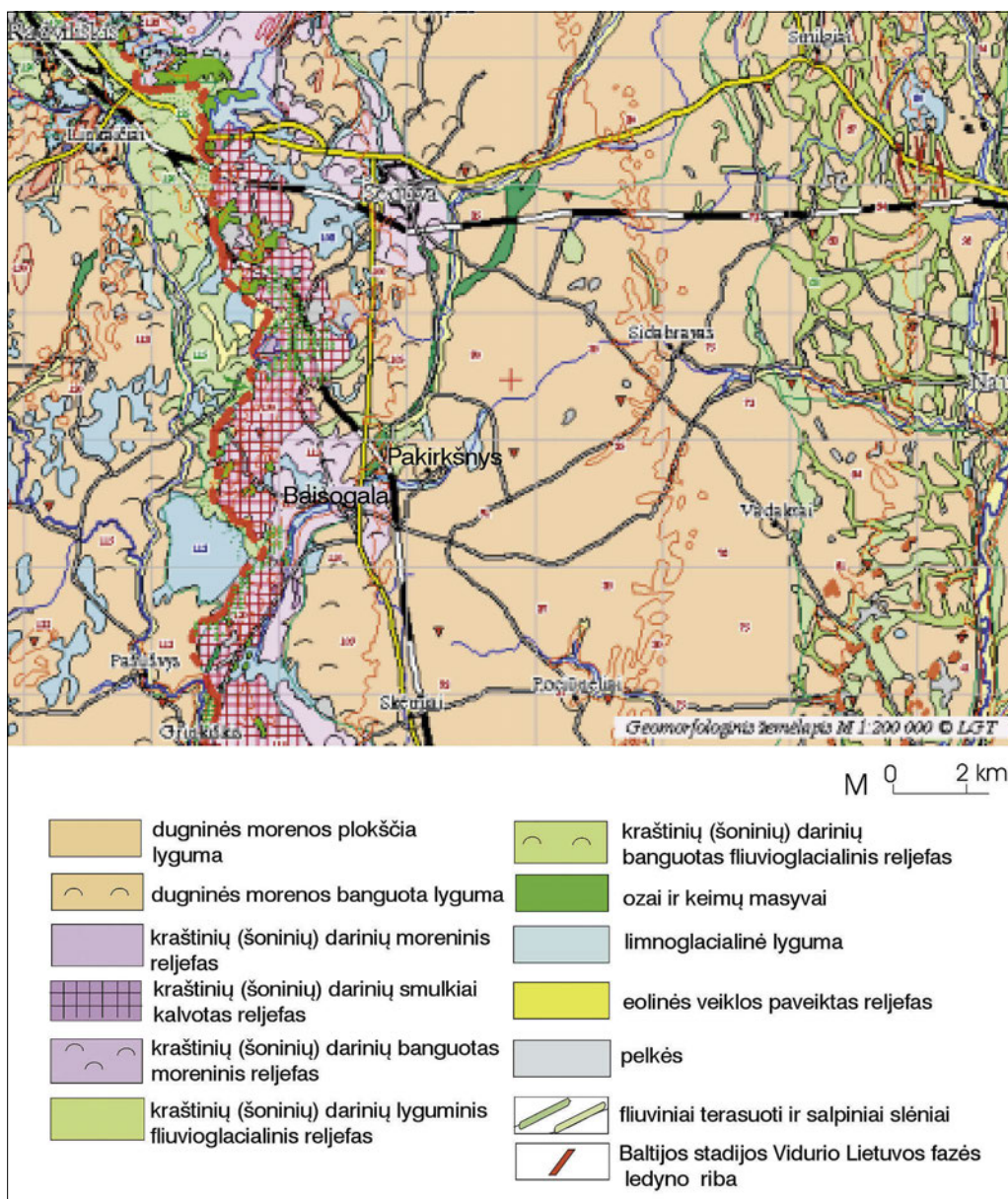
2 pav. Geomorfologinis žemėlapis
