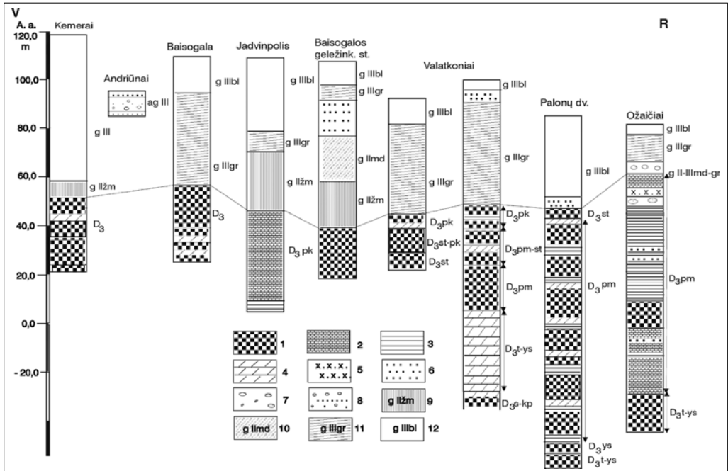
6 pav. Geologinis pjūvis iš vakarų į rytus (Kemeraai, Baisogala, Jadvinpolis, Valatkoniai, Palonų dv., Ožaičiai): 1 – devono sistemos viršutinio skyriaus dolomitai: D_{3s-kp} – Suosos–Kupiškio svitų, D_{3t-ys} – Tatulos–Įstro svitų, D_{3ys} – Ystro svitos, D_{3pm} – Pamūšio svitos, D_{3st-pk} – Stipinų–Pakruojo svitų, D_{3pk} – Pakruojo svitos; 2 – devono sistemos viršutinio skyriaus stipriai plyšiuoti dolomitai: D_{3pm} – Pamūšio svitos, D_{3pk} – Pakruojo svitos; 3 – devono sistemos viršutinio skyriaus moliai: D_{3t-ys} – Tatulos–Įstro svitų, D_{3pm} – Pamūšio svitos, D_{3pk} – Pakruojo svitos; 4 – devono sistemos viršutinio skyriaus mergeliai: D_{3t-ys} – Tatulos–Įstro svitų, D_{3pm-st} – Pamūšio–Stipinų svitų, D_{3pm} – Pamūšio svitos, D_{3pk} – Pakruojo svitos; 5 – devono sistemos viršutinio skyriaus smiltainiai: D_{3pm} – Pamūšio svitos; 6 – devono sistemos viršutinio skyriaus smėliai: D_{3pm} – Pamūšio svitos; 7 – devono sistemos viršutinio skyriaus gargždas: D_{3pm} – Pamūšio svita; kvartero nuogulos: 8 – smėlingos žvirgždingos nuogulos, 9 – vidurinio pleistoceno Žemaitijos apledėjimo morena, 10 – vidurinio pleistoceno Medininkų apledėjimo morena, 11 – viršutinio pleistoceno Nemuno apledėjimo Grūdės stadijos morena, 12 – viršutinio pleistoceno Nemuno apledėjimo Baltijos stadijos morena. Grėžinių išdėstymo schemą žr. 5 pav.
