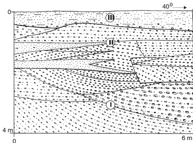
7 pav. Januškoniu karjeras. Kutenos upės terasos nuogulų pjūvis: I – neprakastas žvirgždo sluoksnis, II – žvirgždo sluoksniai ir lizės su įvairiagrūdžio smėlio lėšiais, III – smulkiagrūdžio smėlis su žvirgždo intarpais. Pagal A. Mikalauską ir L. Mikutiene, 1971
