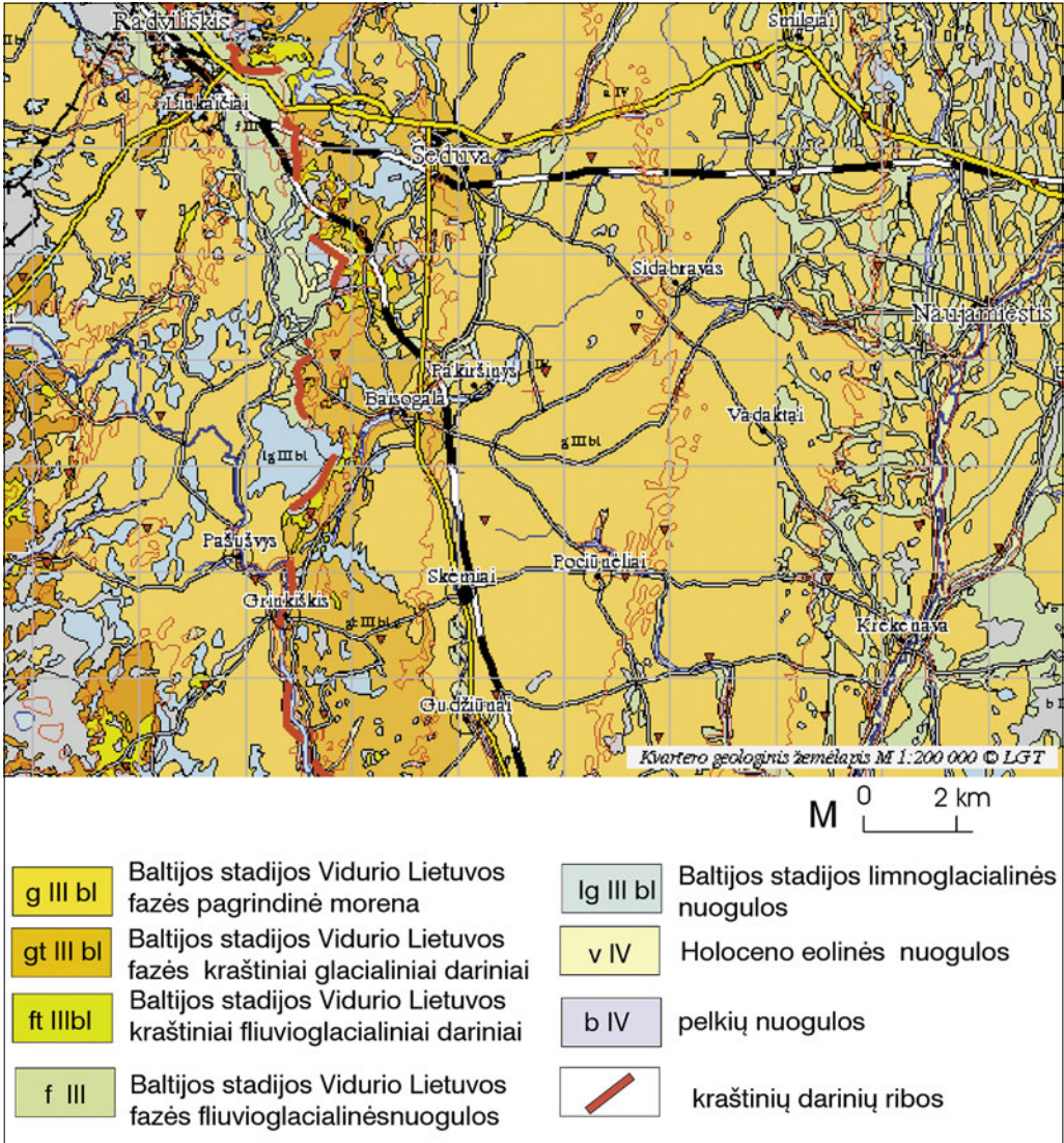
3 pav. Kvartero geologinis žemėlapis
