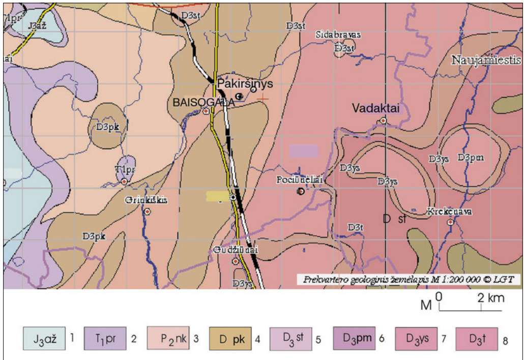
4 pav. Prekvarterio geologinis žemėlapis:
